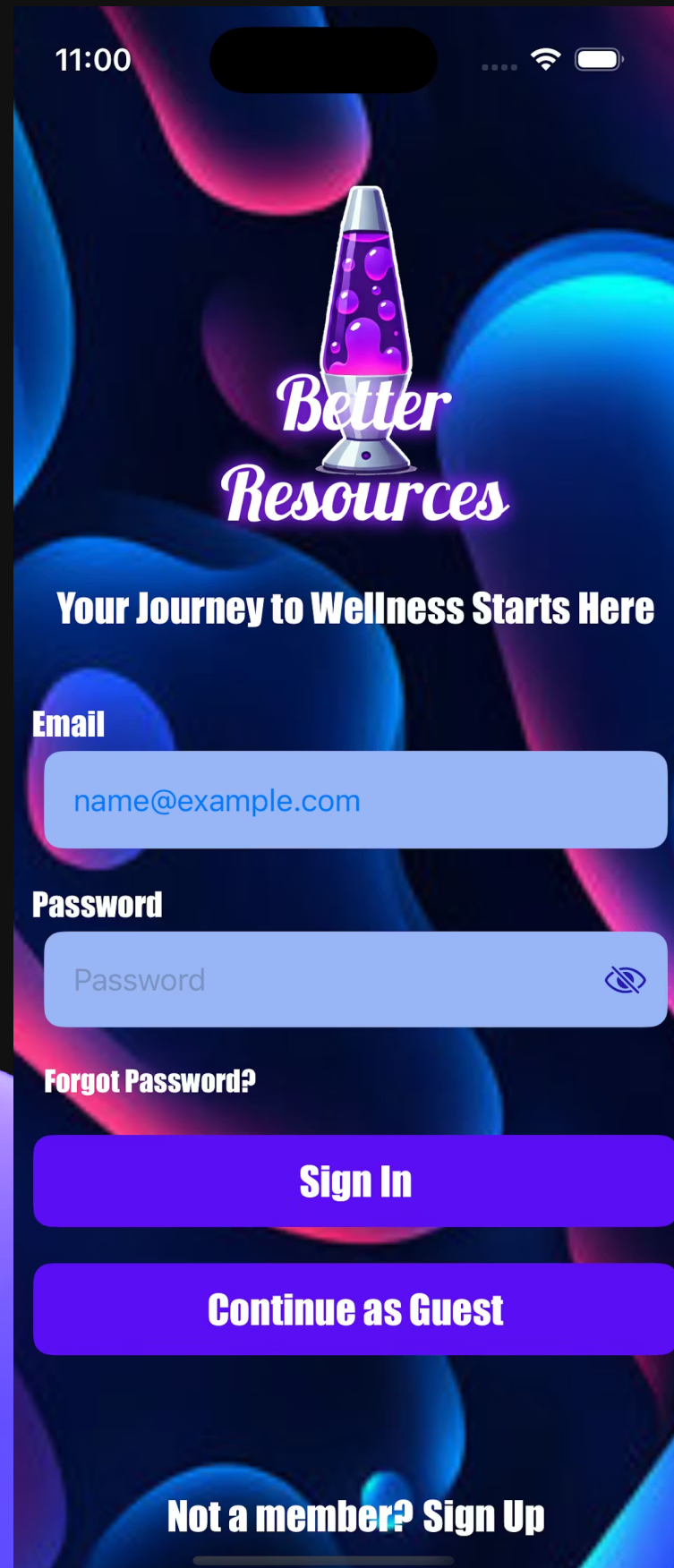
Login Page
